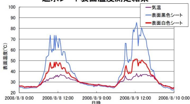
遮水シート表面温度測定結果
